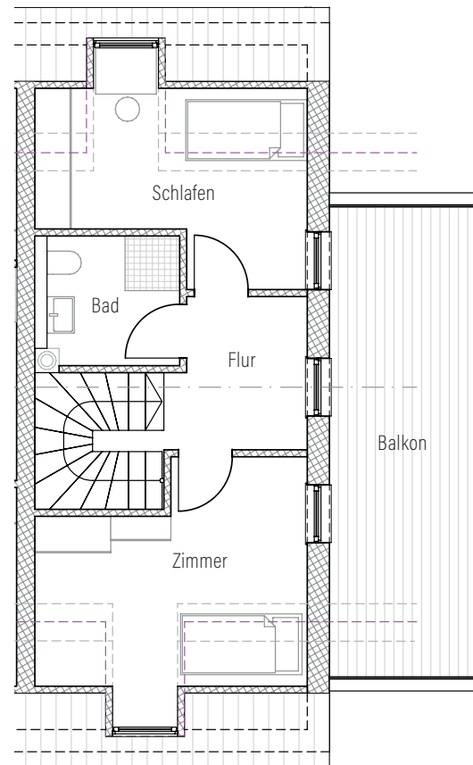
Dachgeschoss
