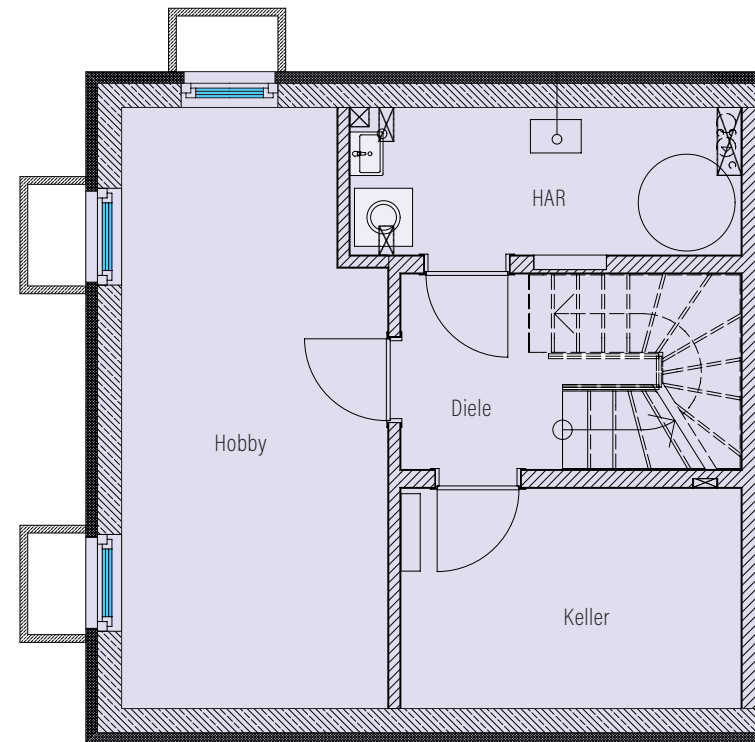
Keller
