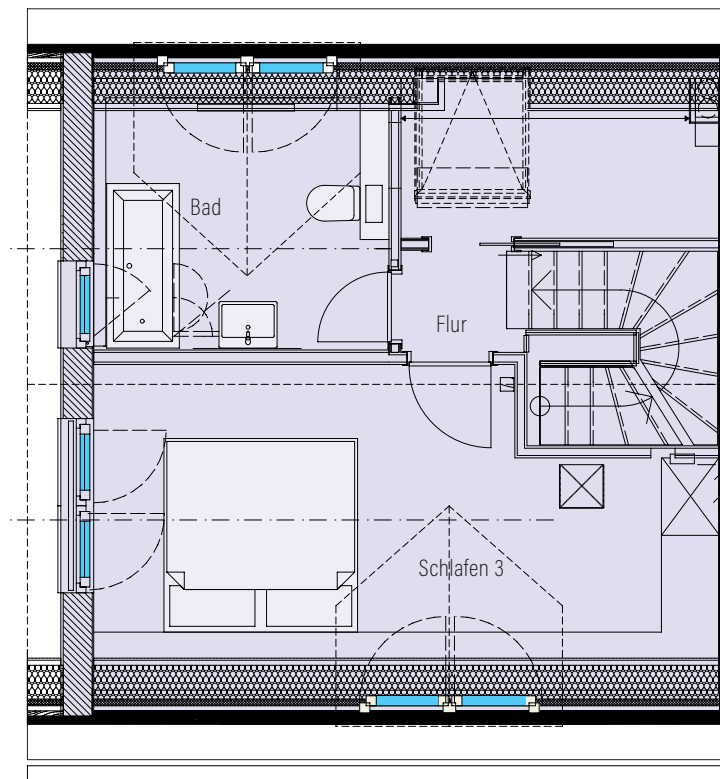
Dachgeschoss
