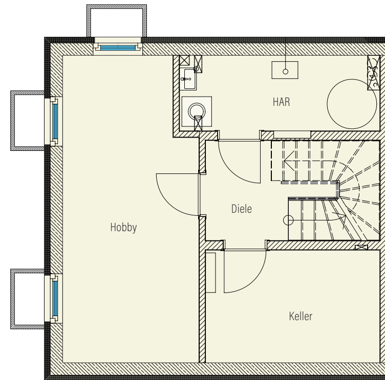
Keller
