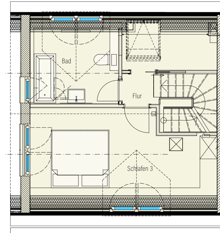
Dachgeschoss
